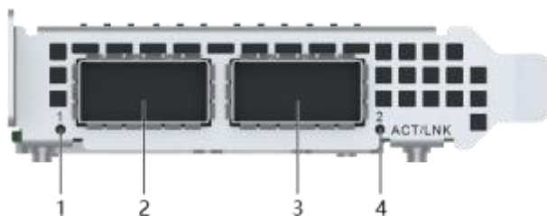
图 1-2 XPU-316 的面板
