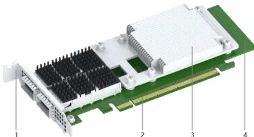
图 1-1 XPU-316的主要部件
